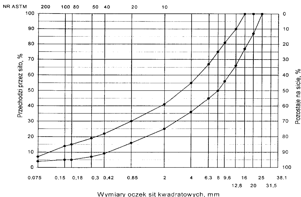
Rys. 2. Krzywe graniczne uziarnienia mieszanek mineralnych BA od 0 do 20 mm do warstwy wiążącej nawierzchni drogi o obciążeniu ruchem KR3
