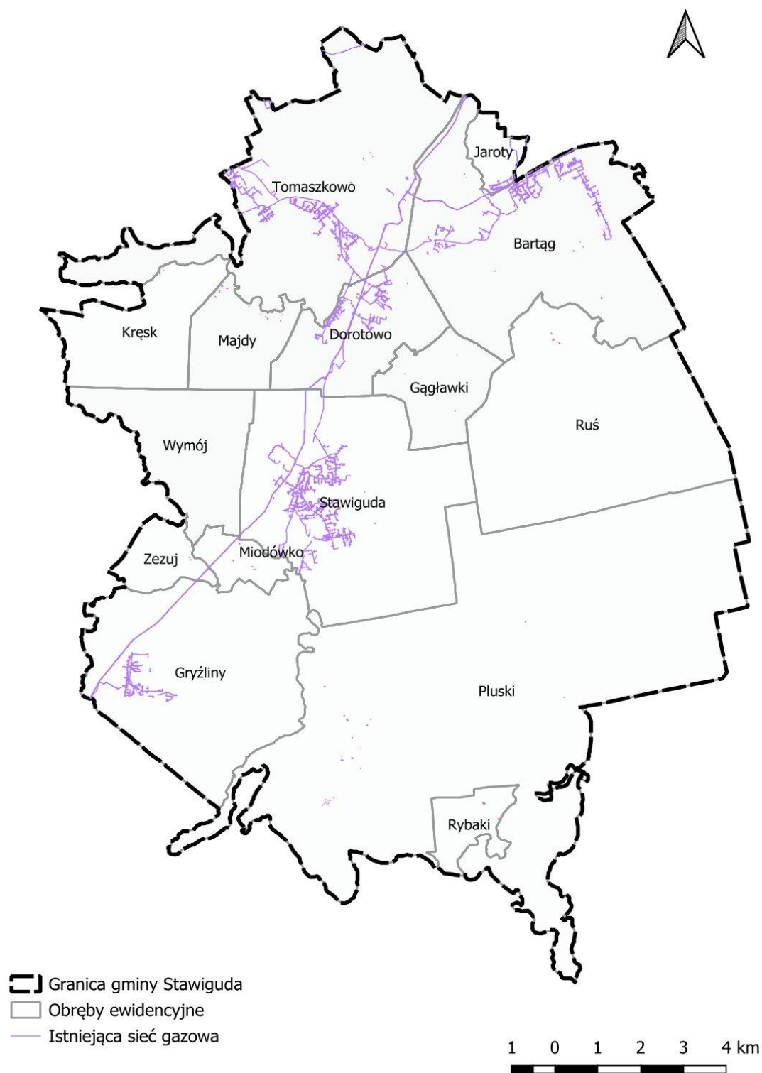
Ryc. 22. Sieć gazowa na terenie gminy Stawiguda
