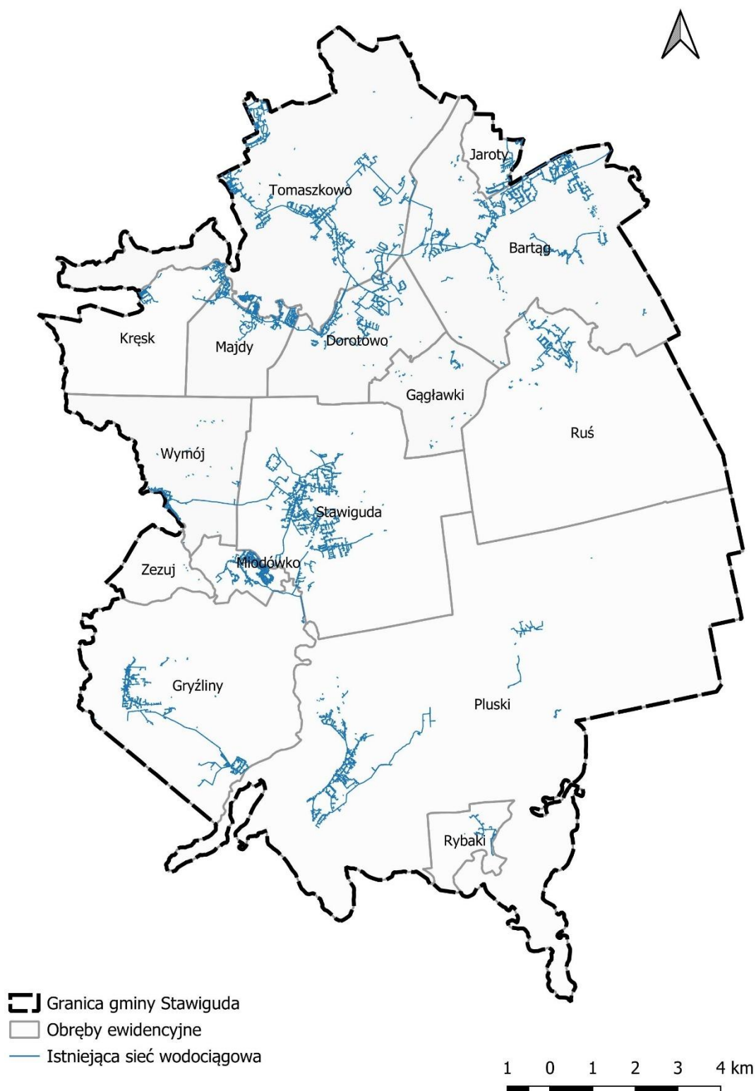
Ryc. 22. Sieć wodociągowa na terenie gminy Stawiguda
