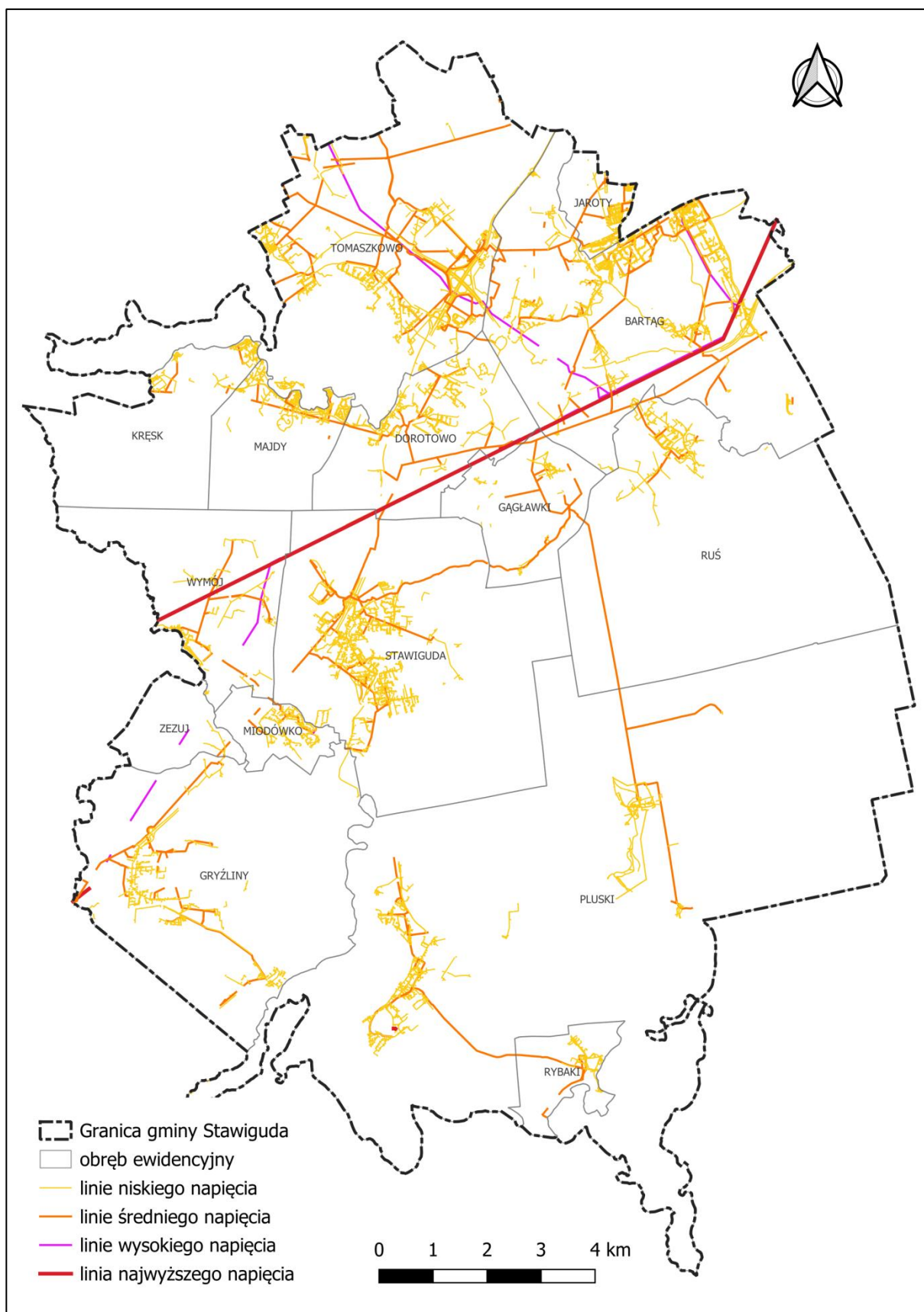
Ryc. 31. Sieć elektroenergetyczna na terenie gminy Stawiguda
