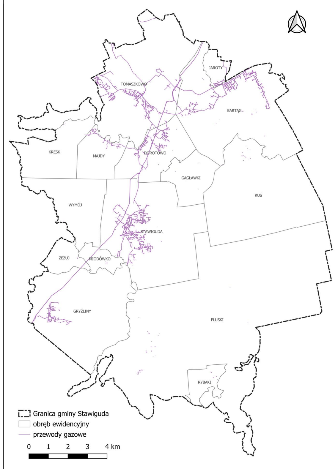
Ryc. 29. Sieć gazowa na terenie gminy Stawiguda
