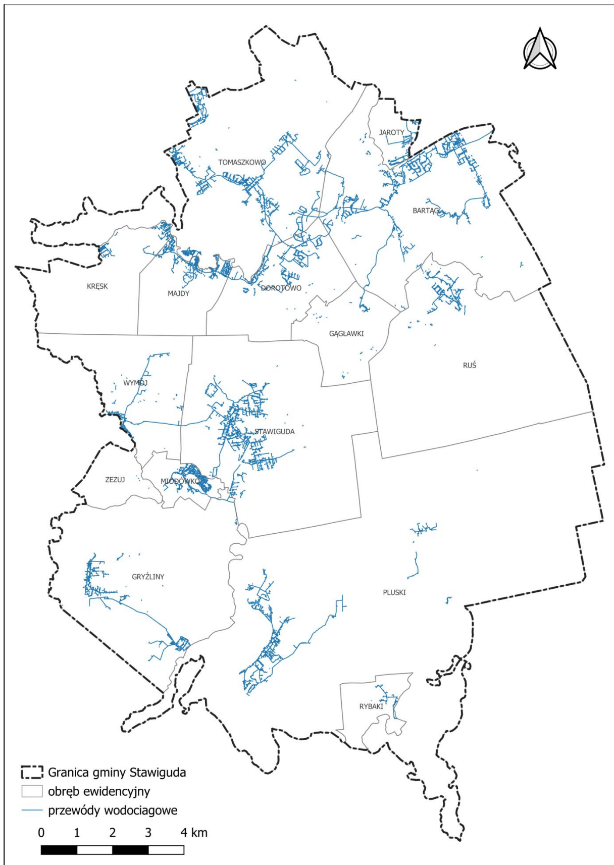
Ryc. 26. Sieć wodociągowa na terenie gminy Stawiguda
