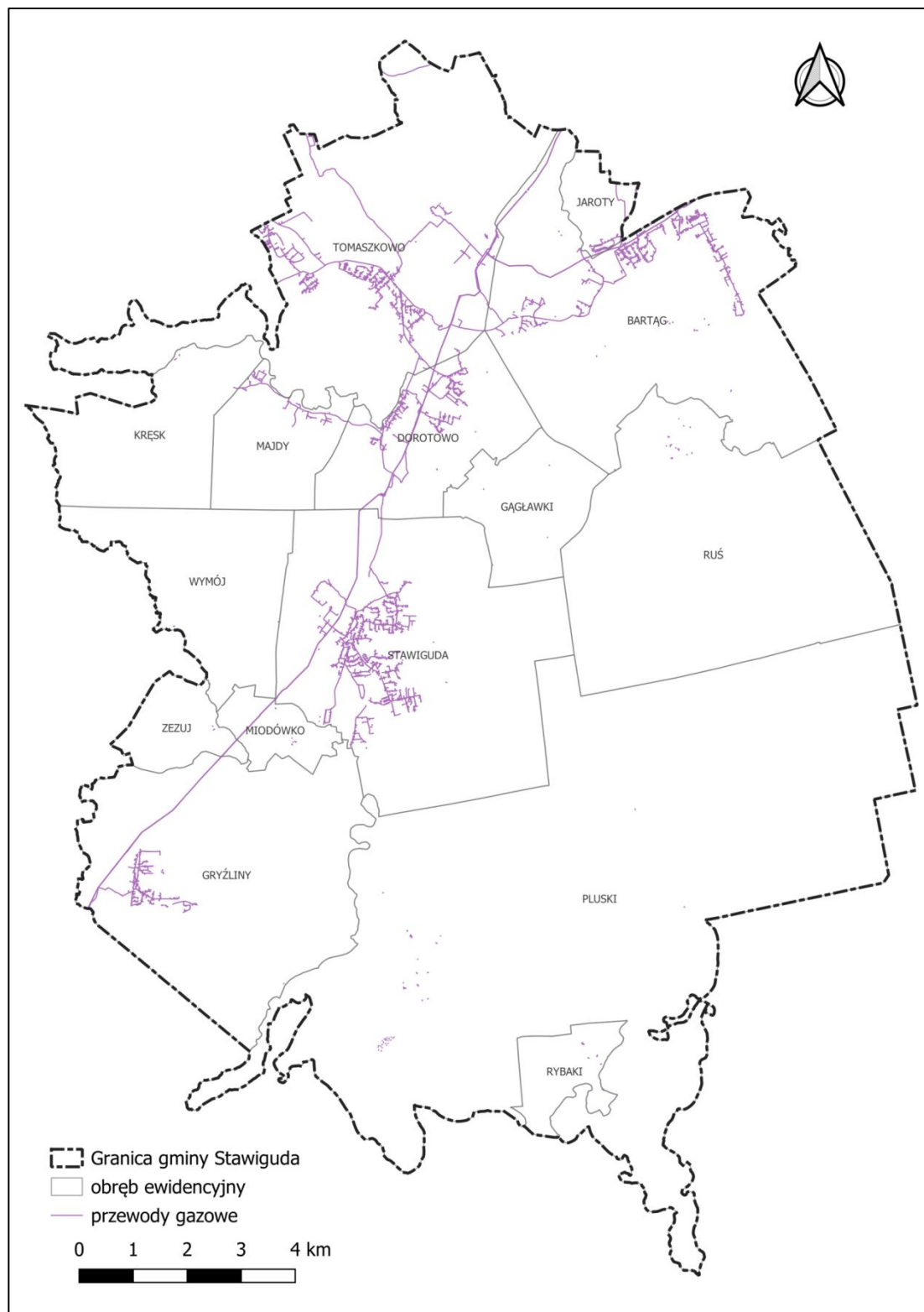
Ryc. 27. Sieć gazowa na terenie gminy Stawiguda
