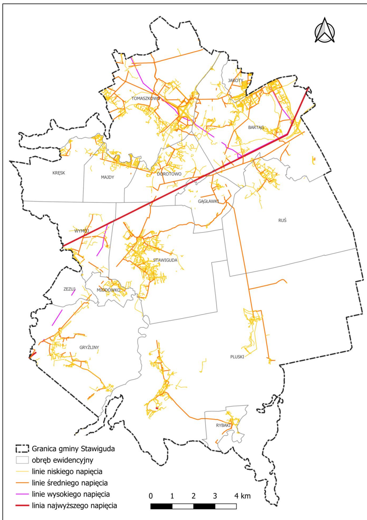
Ryc. 29. Sieć elektroenergetyczna na terenie gminy Stawiguda
