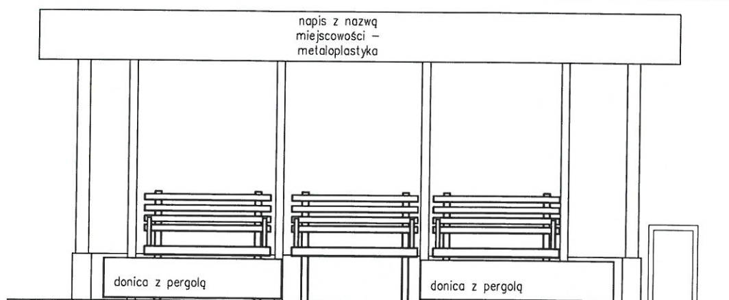
ELEWACJA FRONTOWA
