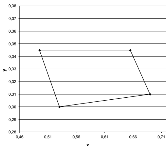
Rys. 1. Współrzędne chromatyczności x, y dla barwy czerwonej oznakowania
