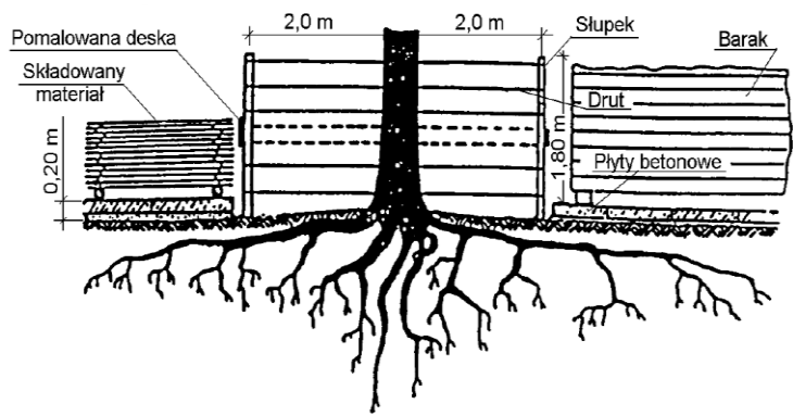
Oprócz wygradzenia drzewa płotem z desek lub żerdzi pokazano z lewej sposób składowania materiału, a z prawej lokalizację baraku budowy.
