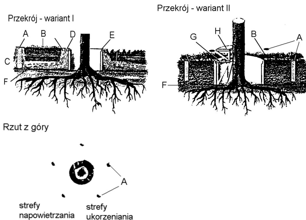
Rys. 5. Studzienka zabezpieczająca pień drzewa przy podwyższeniu terenu powyżej 0,5 m
