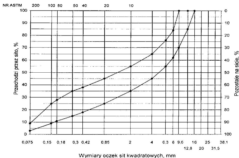
Rys. 10. Krzywe graniczne uziarnienia mieszanki mineralnej BA od 0 do 12,8 mm do warstwy wiążącej, wyrównawczej i wzmacniającej nawierzchni drogi o obciążeniu ruchem KR2
