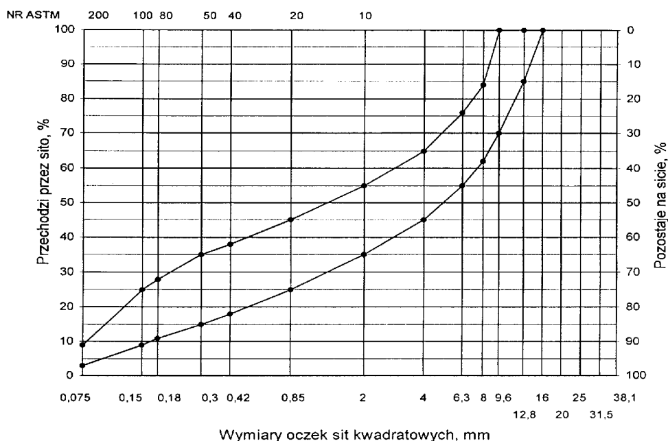
Rys. 9. Krzywe graniczne uziarnienia mieszanki mineralnej BA od 0 do 16 mm do warstwy wiążącej, wyrównawczej i wzmacniającej nawierzchni drogi o obciążeniu ruchem KR2
