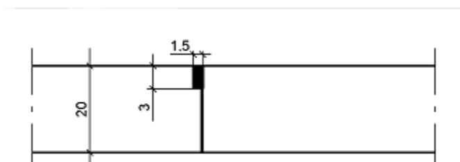
Rys. 1.1. Przykłady konstrukcji szczelin w podbudowie z betonu cementowego (wymiary w cm)
