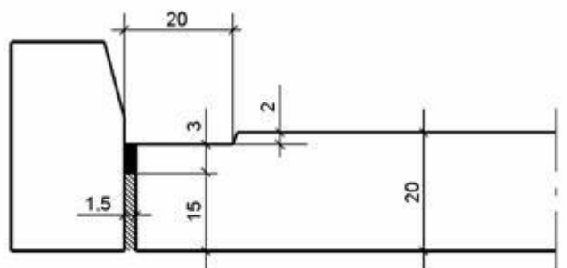
Szczelina nacięta w podbudowie (bez wypełnienia), na której będzie ułożona warstwa ścierna z mieszanki mineralno-asfaltowej
