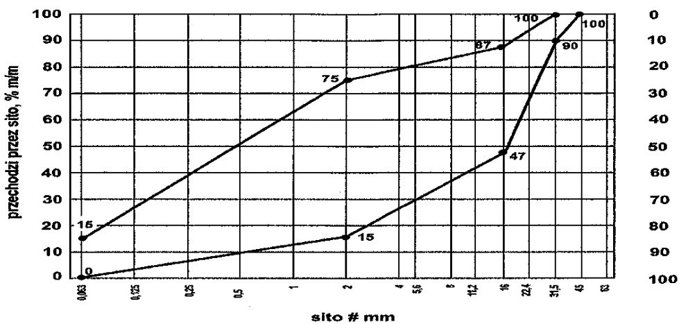
Rys. 5. Krzywe graniczne uziarnienia mieszanki kruszyw 0/31,5 mm do górnej warstwy podłoża ulepszzonego
