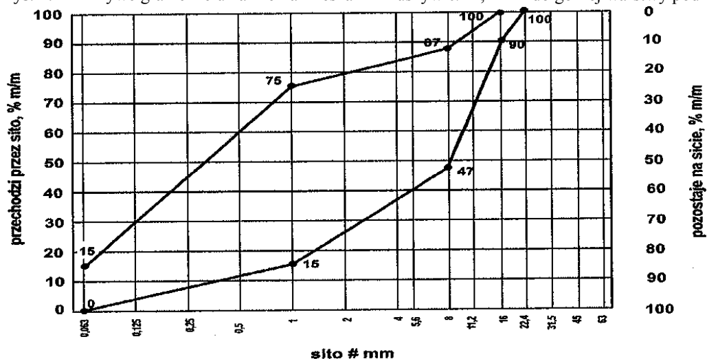
Rys. 2. Krzywe graniczne uziarnienia mieszanki kruszyw 0/11,2 mm do górnej warstwy podłoża ulepszzonego
