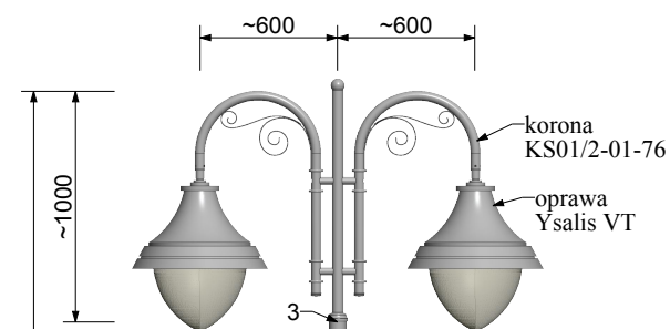
POŁĄCZENIE LATARNI Z KORONĄ 3
