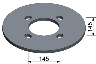
PODSTAWA 1
