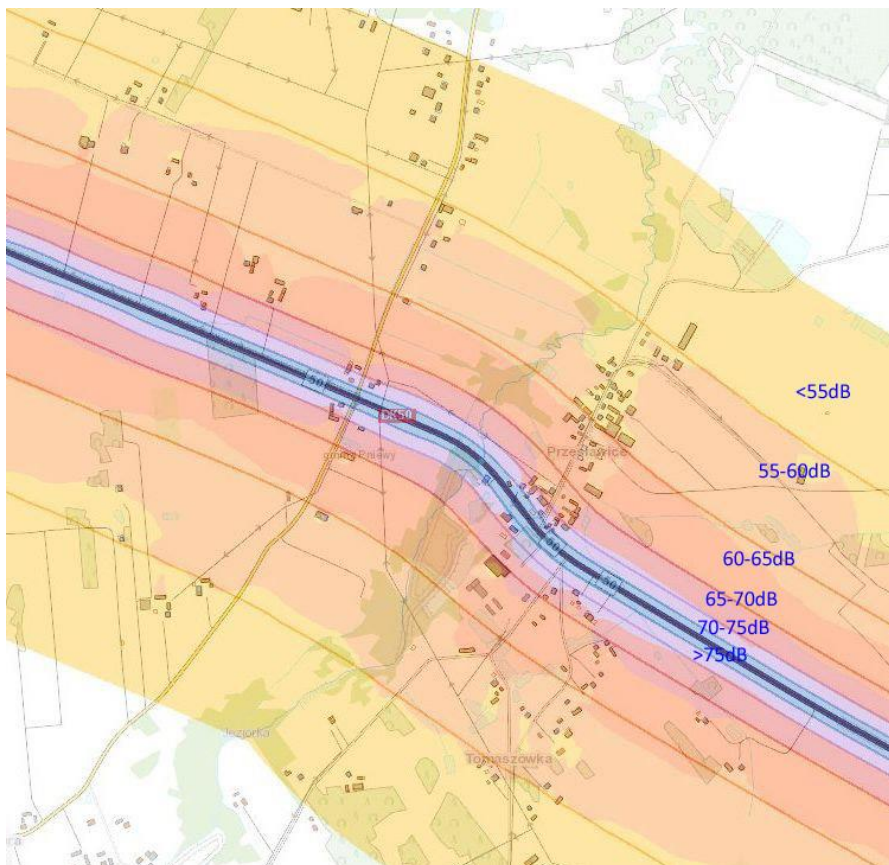
Rysunek 10 Mapa akustyczna wyrażona wskaźnikiem LDWN odcinka DK50 w miejscowości Przęgławice
