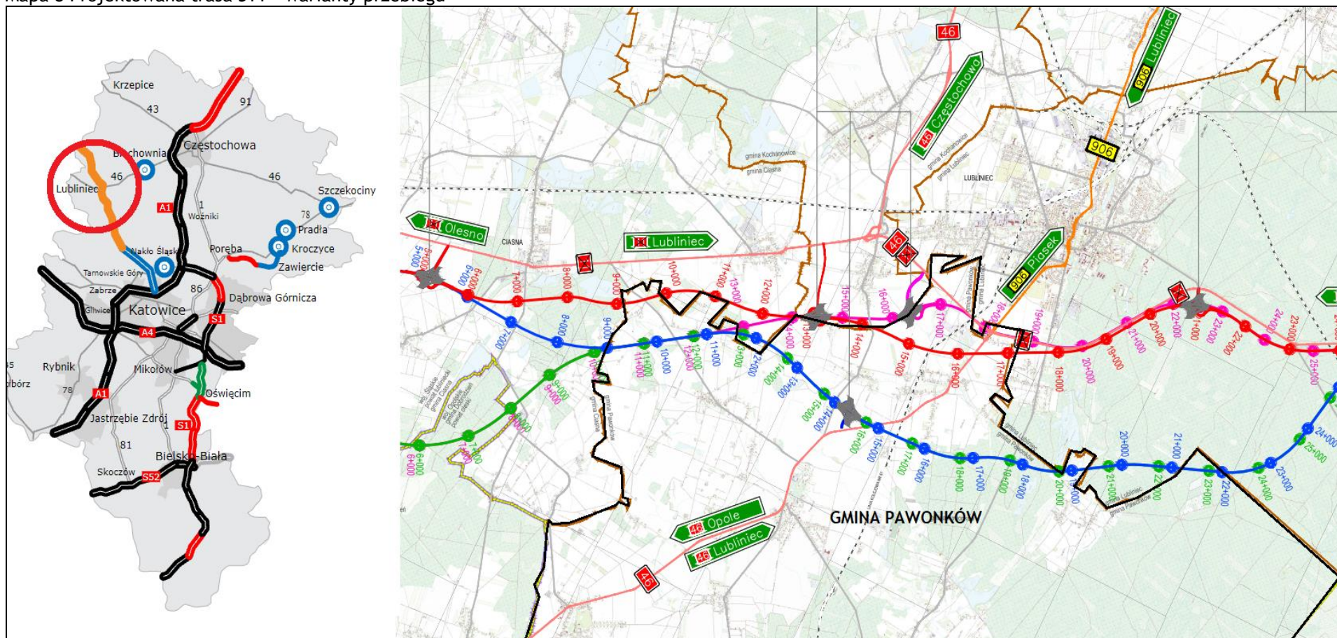
Mapa 8 Projektowana trasa S11 - warianty przebiegu
