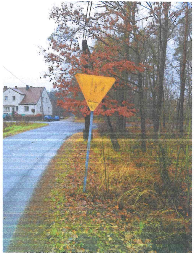
Znak A-7 "ustąp pierwszeństwa" (skrzyżowanie ul. Szkolnej z drogą powiatową 2321 S) Znak nie jest widoczny w nocy, słabo odbija światło.
