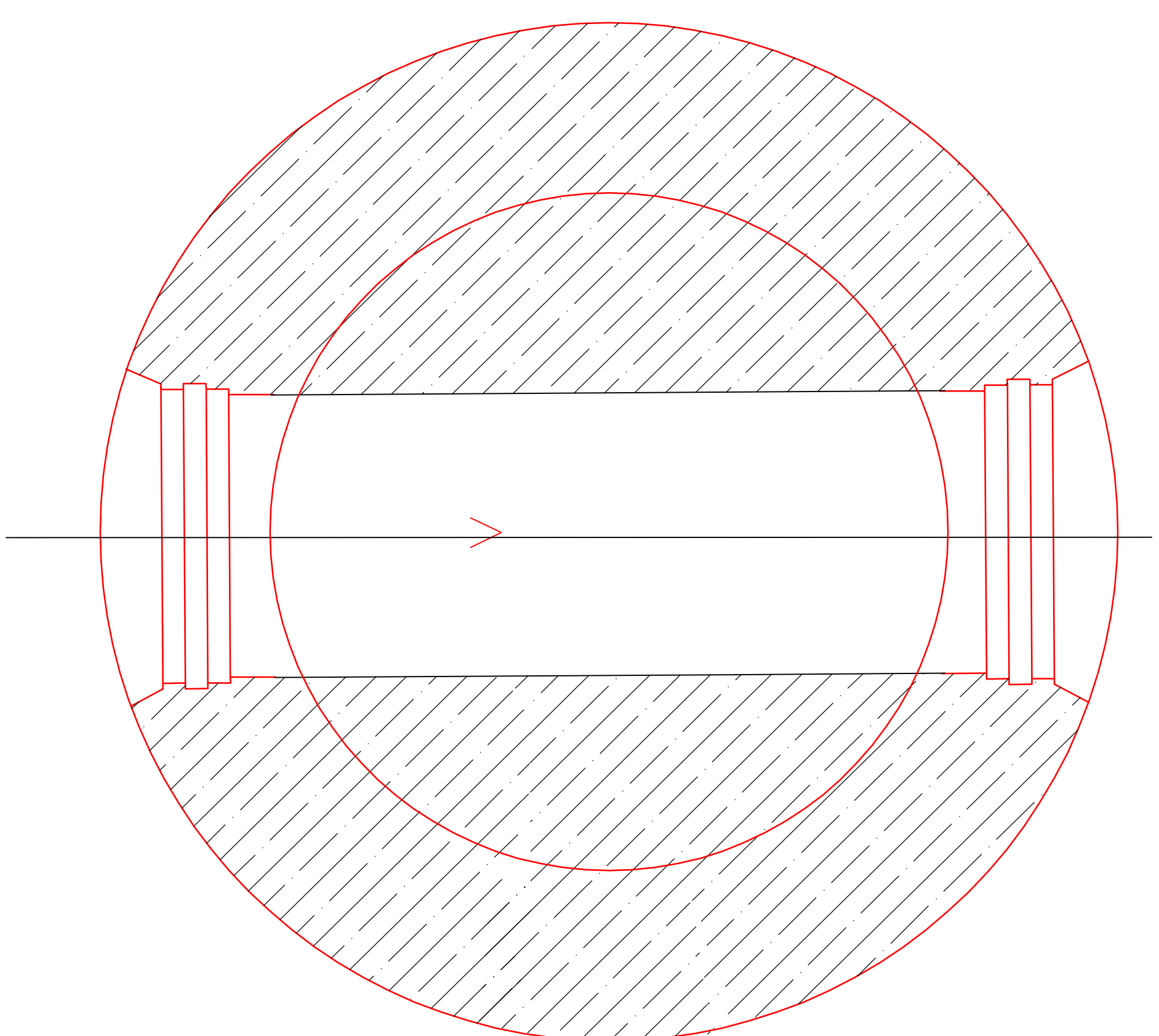
Dno Studni z wyprofilowaną kinetą
