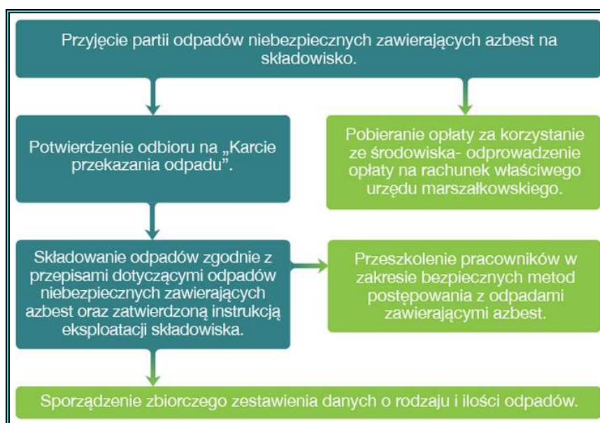
Ryc. 9. Procedura 6 - dotycząca składowania odpadów na składowisku przeznaczonym do wyłącznego składowania odpadów zawierających azbest lub innym, spełniającym odpowiednie warunki techniczne
