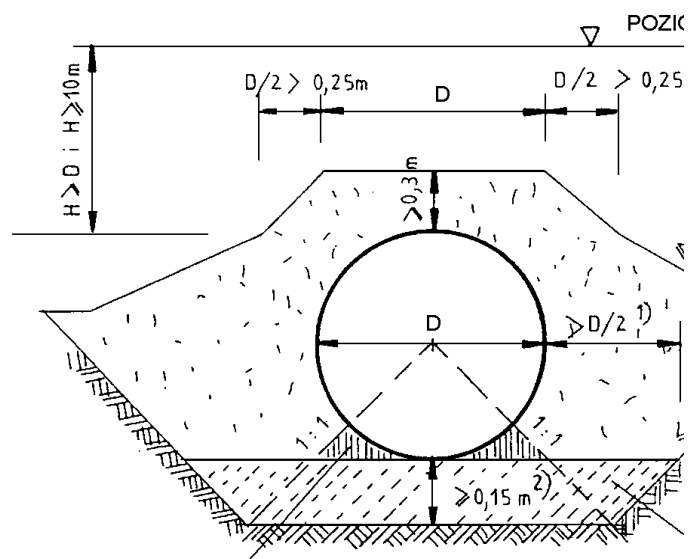
Rys. 9. Zasyпка nad przepustem dwururowym
