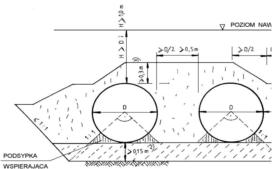
Rys. 10. Przykład umocnienia skarpy przy wlocie przepustu za pomocą drobnowymiarowych elementów z betonowej kostki brukowej lub kamienia
