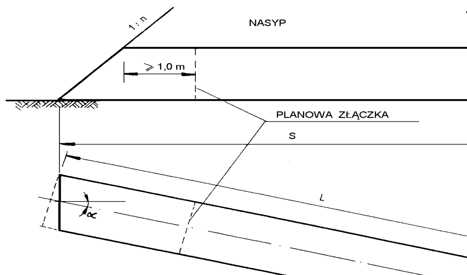
Rys. 7. Końcowy, skrajny odcinek rury nie powinien być krótszy od 1 m
