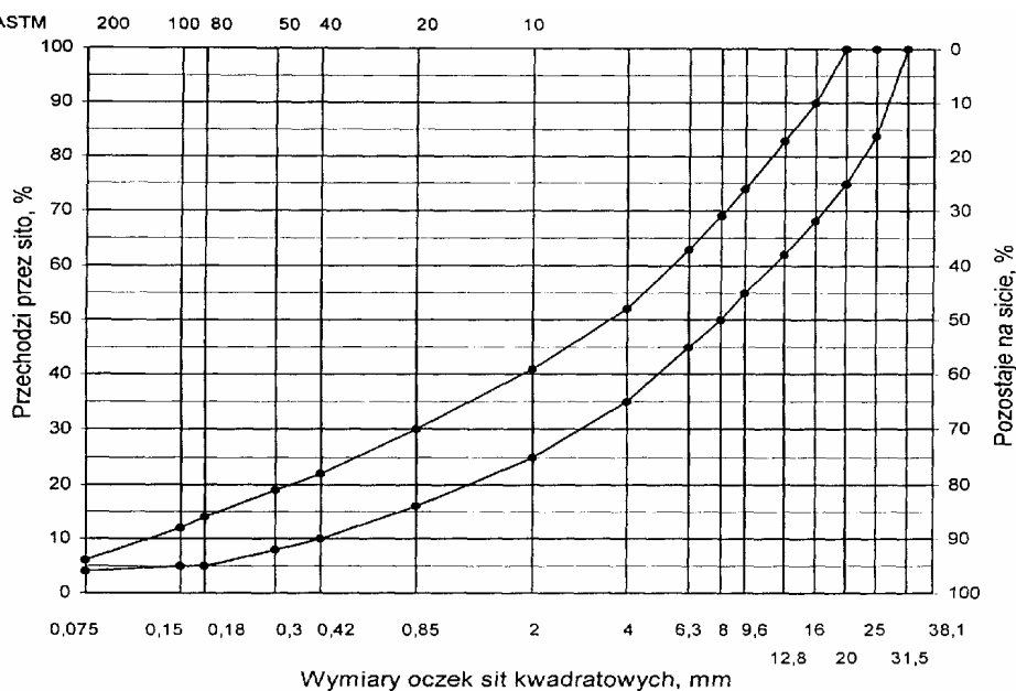
Rys. 11. Krzywe graniczne uziarnienia mieszanki mineralnej BA od 0 do 25 mm do warstwy wiążącej nawierzchni drogi o obciążeniu ruchem od KR3 do KR6
