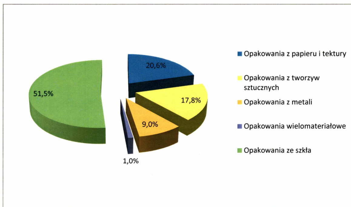
Rysunek 6. Masa odpadów komunalnych poddana recyklingowi w 2018 r. [%]
