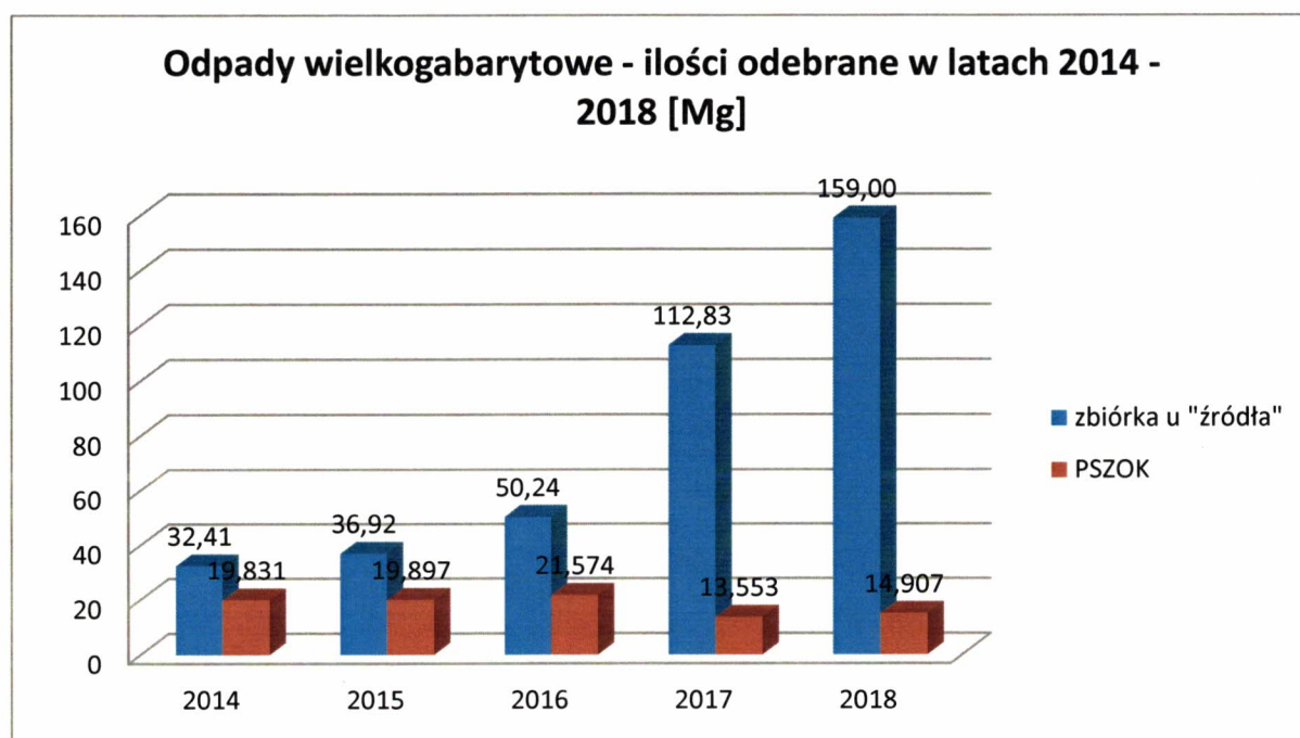
Rysunek 5. Masa odpadów wielkogabarytowych pochodząca z nieruchomości objętych gminnym systemem gospodarki odpadami, odebrana i zebrana w latach 2014 - 2018
