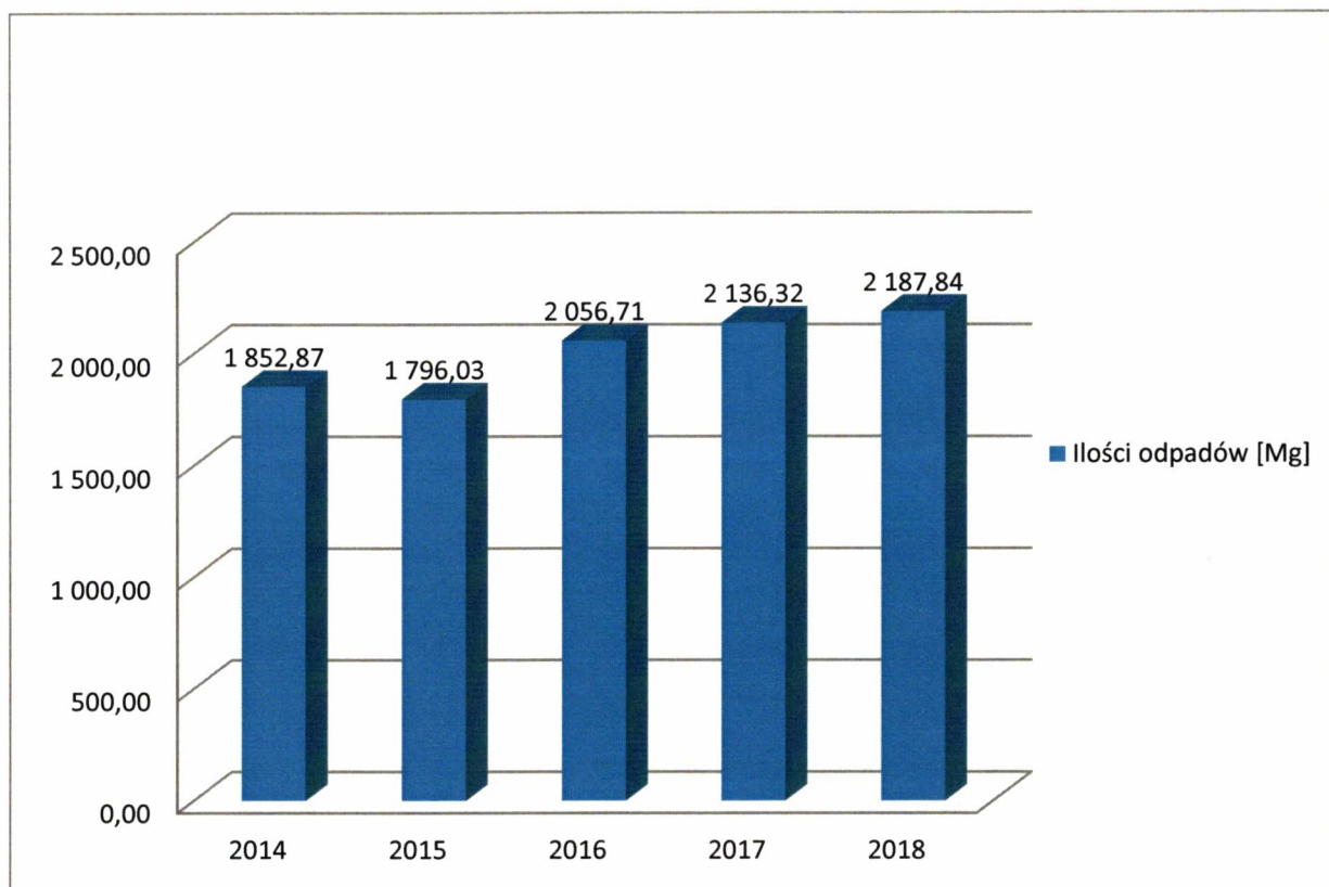
Rysunek 4. Zmieszane (mokre) odpady komunalne odebrane z nieruchomości objętych gminnym systemem gospodarki odpadami
