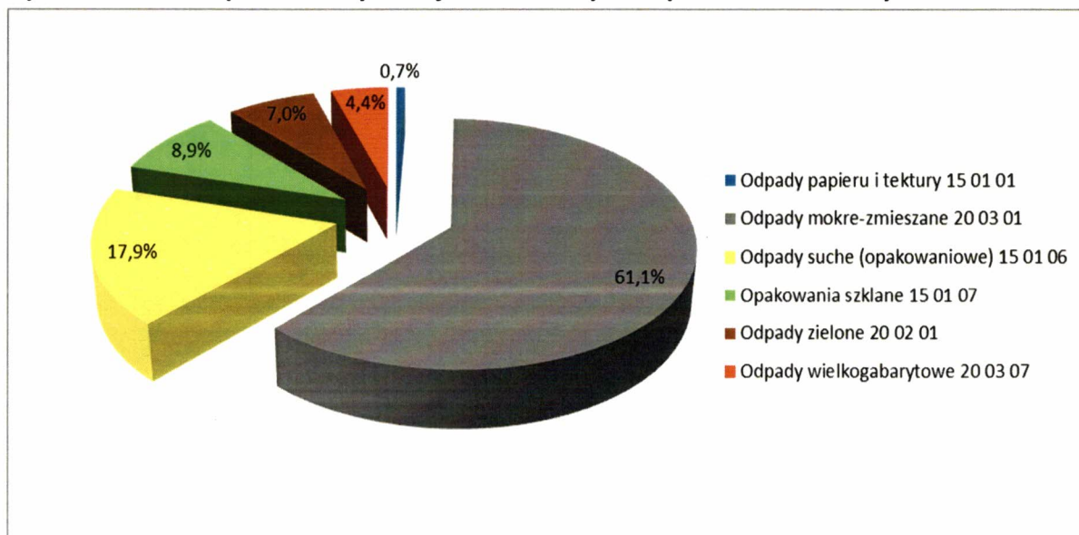
Rysunek 3. Udział procentowy frakcji w odebranych odpadach komunalnych
