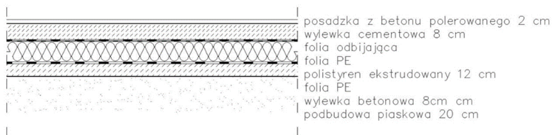
P2 (detal 4 1:20)
