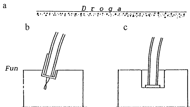
Załącznik 11 Przykład połączenia śrubami blach falistych 1 - śruba M 20 2 - nakrętka M
