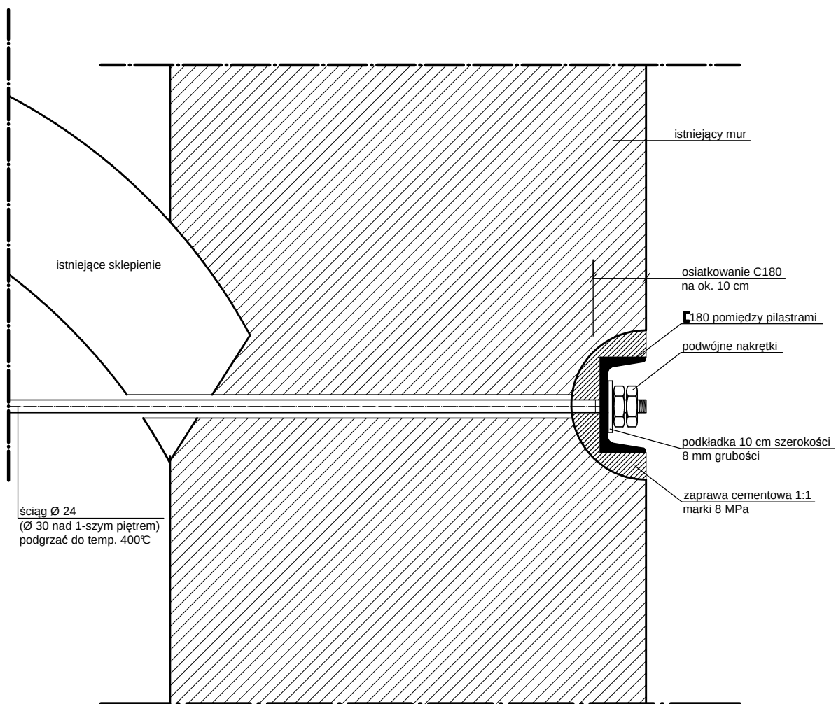
Szczegół skotwienia wychylonych z pionu ścian zewnętrznych oraz wzmocnienia ściągi stalowymi sklepień
