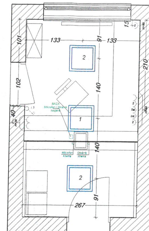
Schemat rozmieszczenia elektryki - pomieszczenie kasowe
