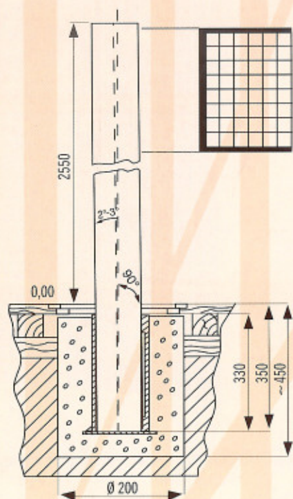
schemat ideowy montażu
