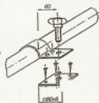
Elementy mocowania bramki do podłogi
