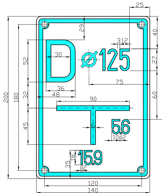
Tablica orientacyjna dla hydrantu PN - 86/B-09700-1
