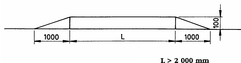
b. Próg płytowy typu 1A 2 w km 0+402 z przejściem pieszym
