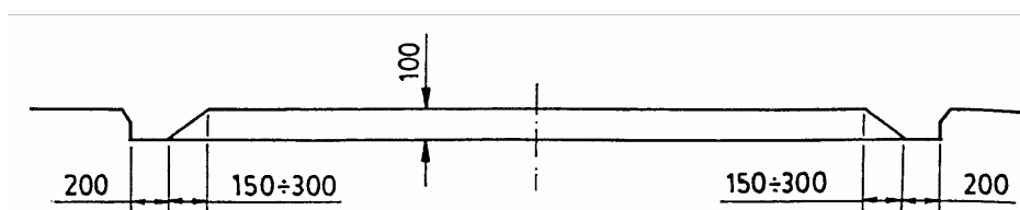
a. Próg listwowy w przekroju poprzecznym jezdni w km 0+402
