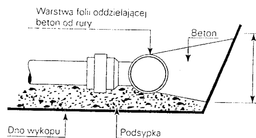
b/ widok z boku
