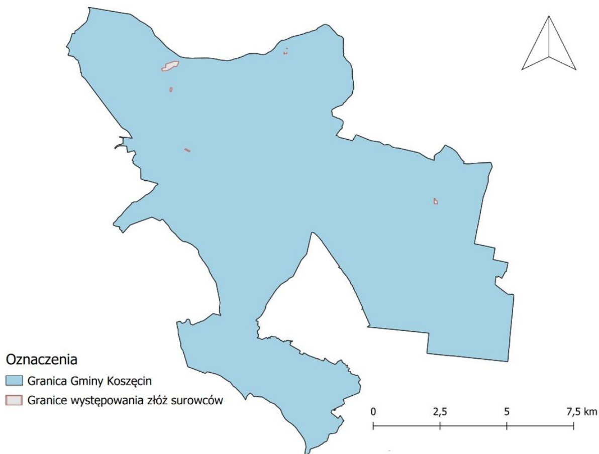
Ryc. 19. Występowanie złóż surowców naturalnych na terenie Gminy Koszęcin
