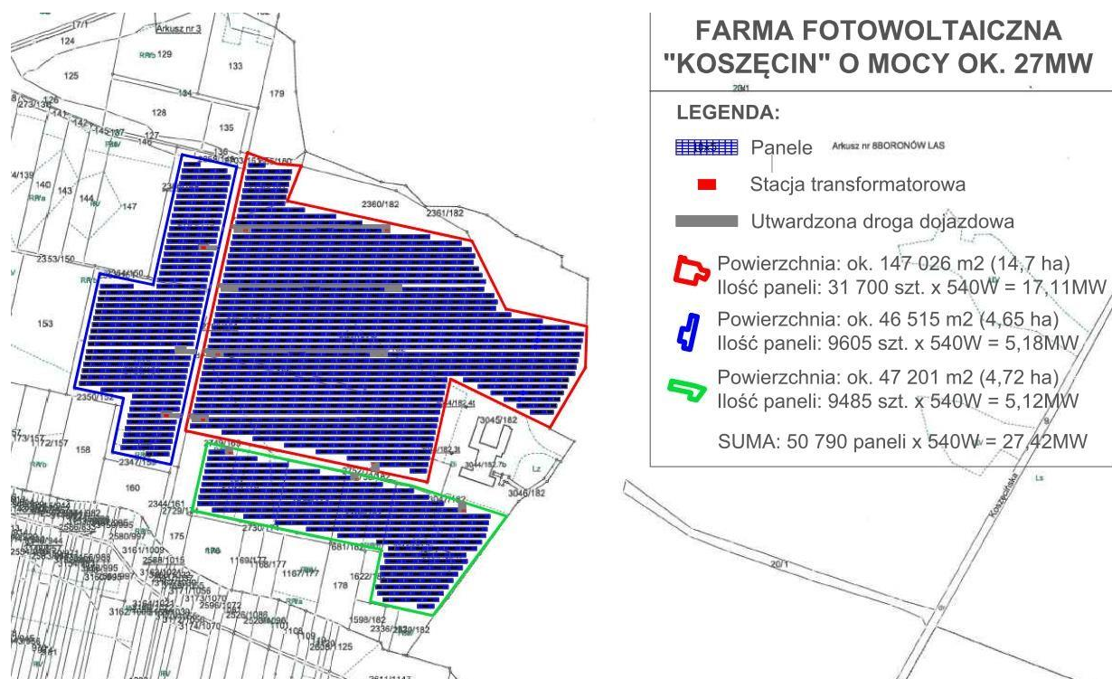
Rysunek 5. Poglądowe rozmieszczenie paneli w granicach działek inwestycyjnych [źródło: materiały inwestora].
