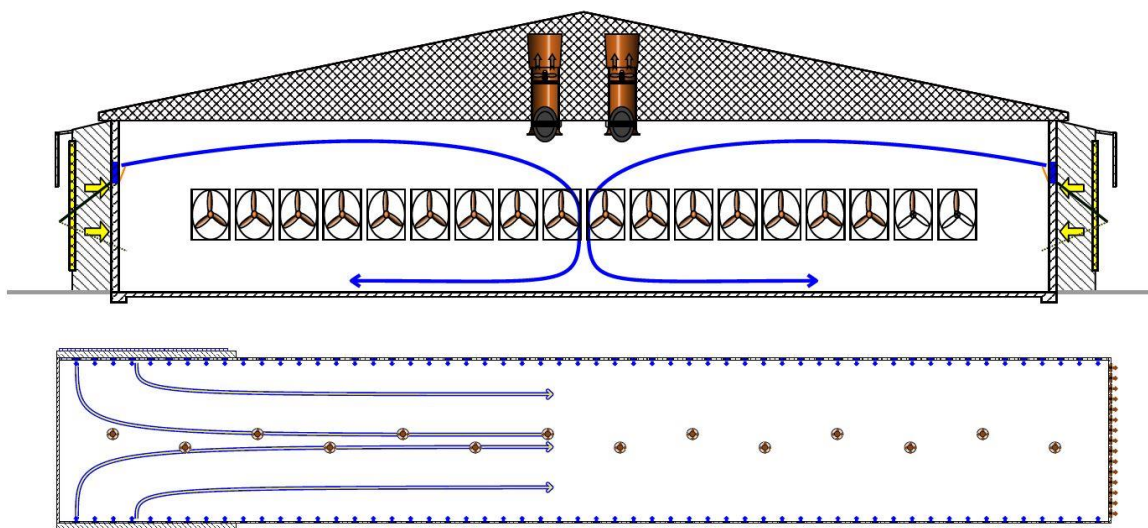
Rys. 10. Poglądowy układ pracy wentylacji (u góry tryb boczny, na dole tunelowy).
