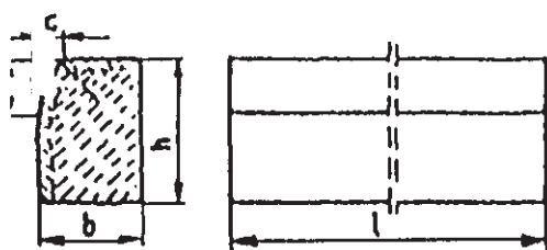
a) krawężnik rodzaju „a”
