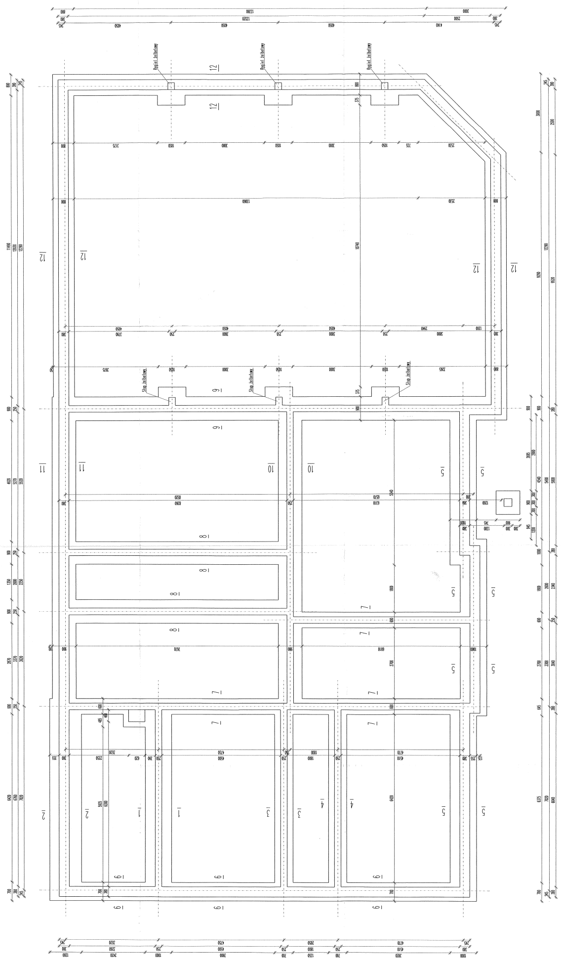
RZUT FUNDAMENTÓW 1:50
