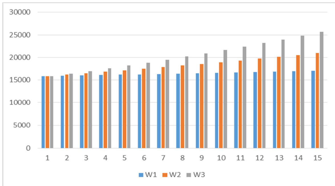
Rysunek 14 Dynamika zapotrzebowania na energię elektryczną do roku 2035
