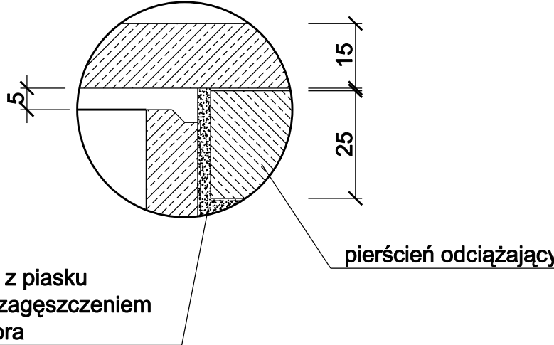
SZCZEGÓŁ "A" 1:25
