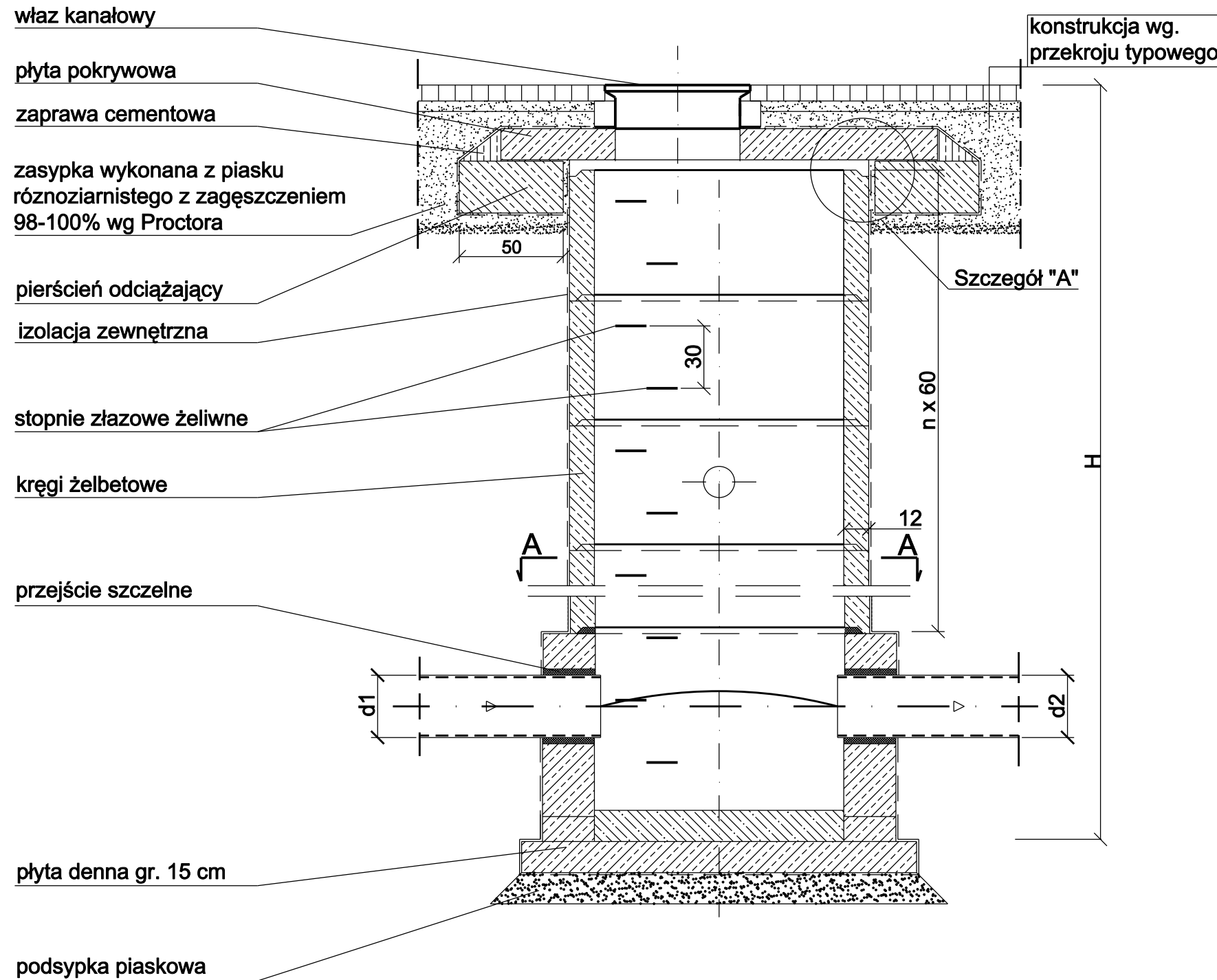
PRZEKRÓJ POPRZECZNY skala 1:50
