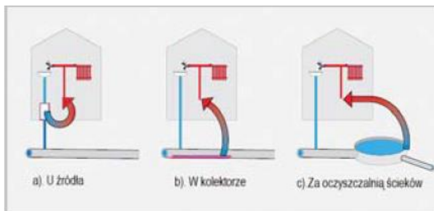
Rysunek 36 Lokalizacja możliwych punktów odbioru ciepła ze ścieków
