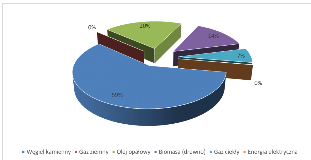
Rysunek 11 Struktura paliwowa pokrycia potrzeb cieplnych gminy Kochanowice[%]
