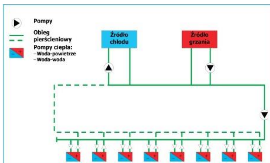
Rysunek 33 Schemat systemu WLHP Źródło: www.chlodnictwoiklimatyzacja.pl
