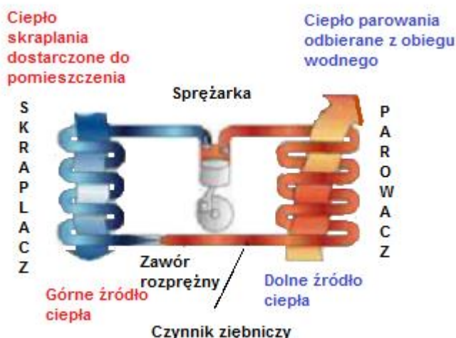
Rysunek 35 Tryb pracy ogrzewania rewersyjnej pompy ciepła Źródło: Lipska B. Wykład- Odzysk energii w wentylacji i klimatyzacji
