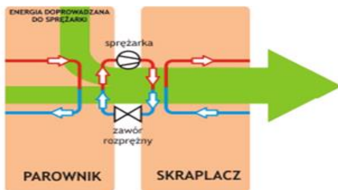
Rysunek 28 Obieg pośredni pompy ciepła, Źródło: Instytut Energetyki Odnawialnej (EC BREC IEO)
