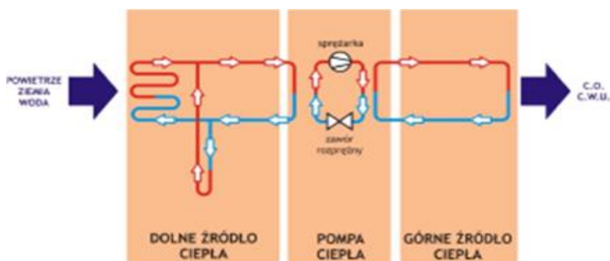
Rysunek 27 Zasada działania pompy ciepła, Źródło: Instytut Energetyki Odnawialnej (EC BREC IEO)
