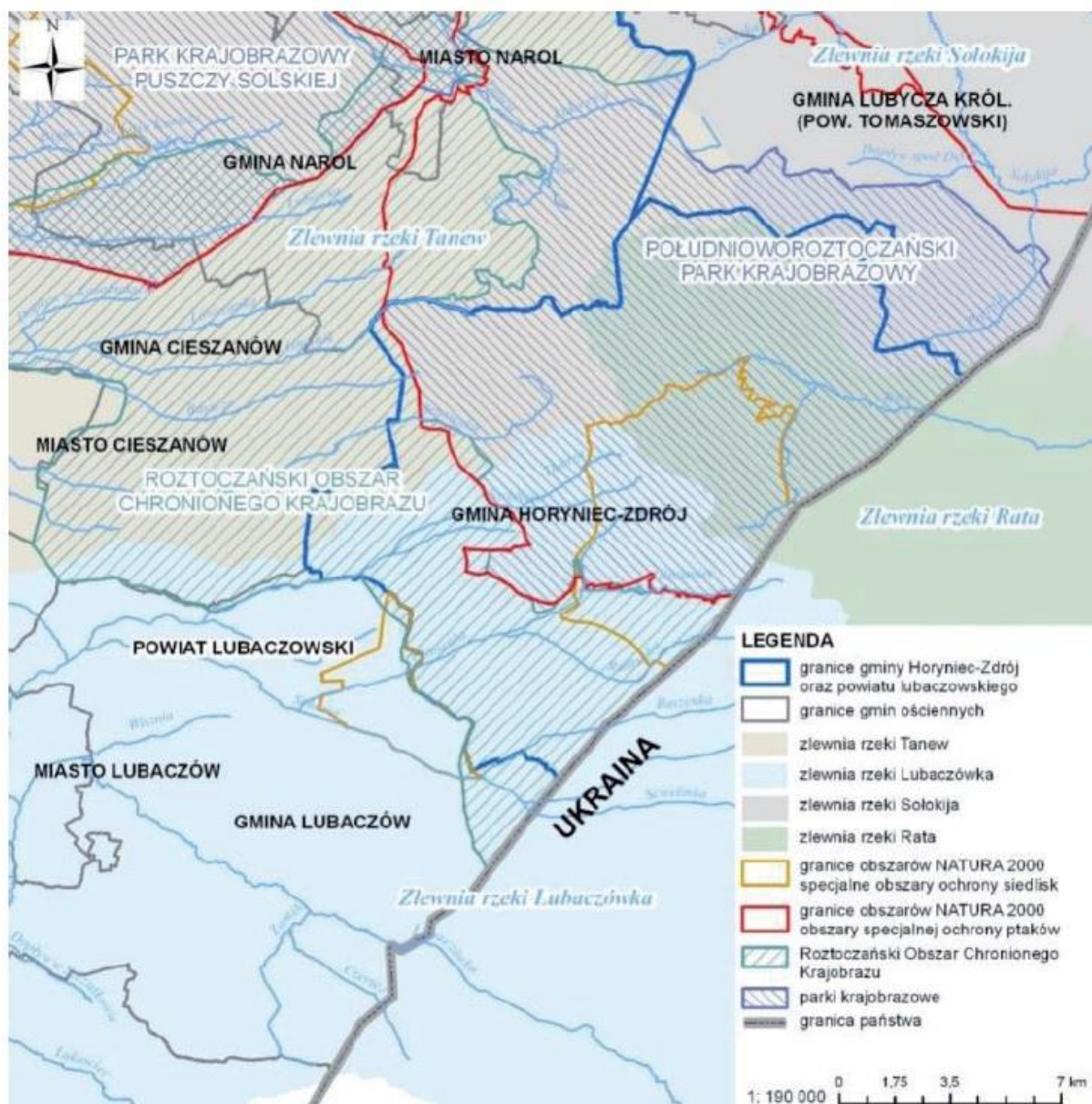
Rysunek 6. Obszar Gminy Horyniec-Zdrój w układzie hydrograficznym.
