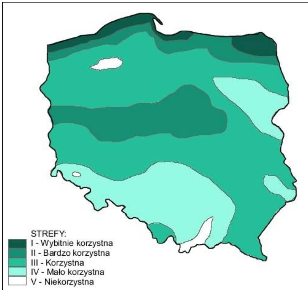
Rysunek 14. Strefy energetyczne warunków wiatrowych.
