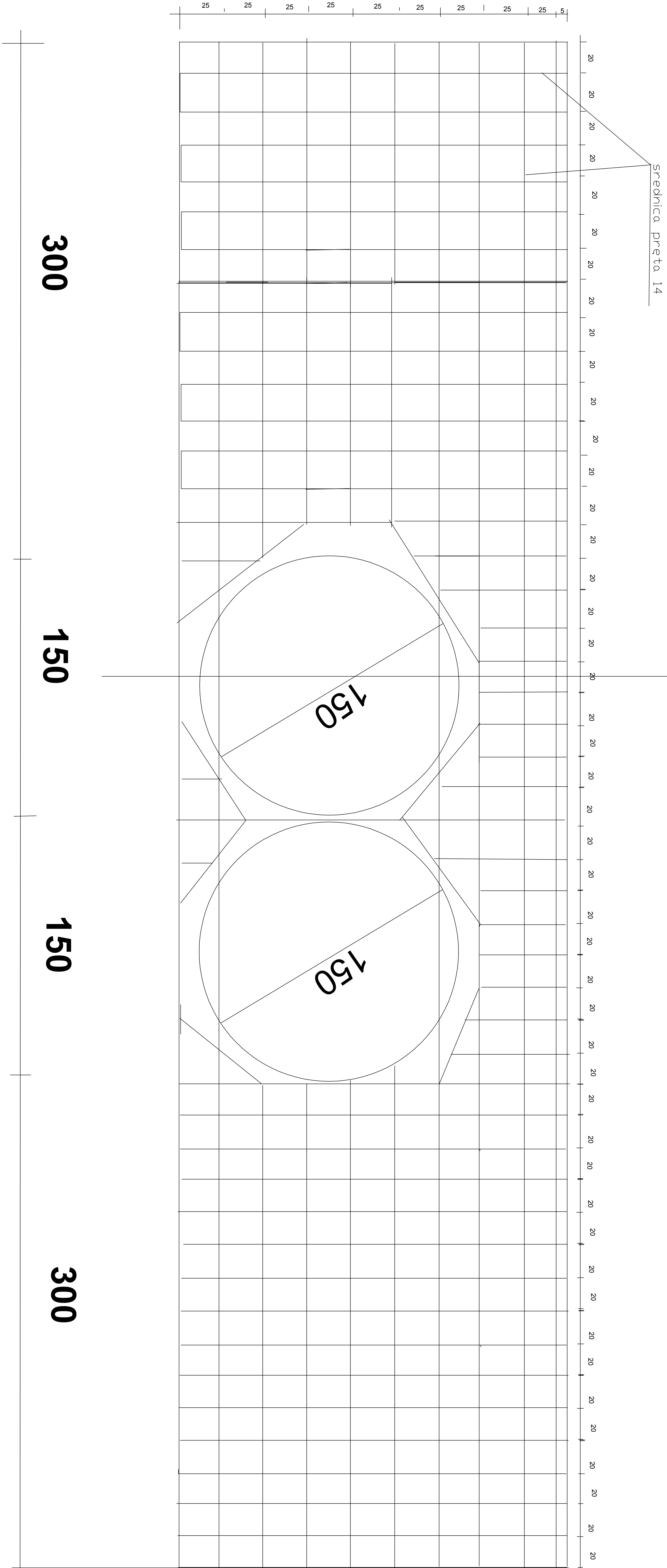
zbrojenie ścianki
