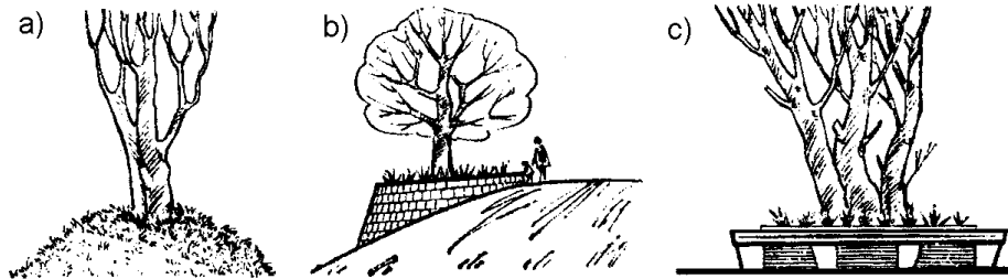
Rys. 2. Zabezpieczenie drzew przy obniżeniu terenu, po wykonaniu wykopów (wg N.P. Omatski: Drogi i ochrona przyrody, Transport 1982)
