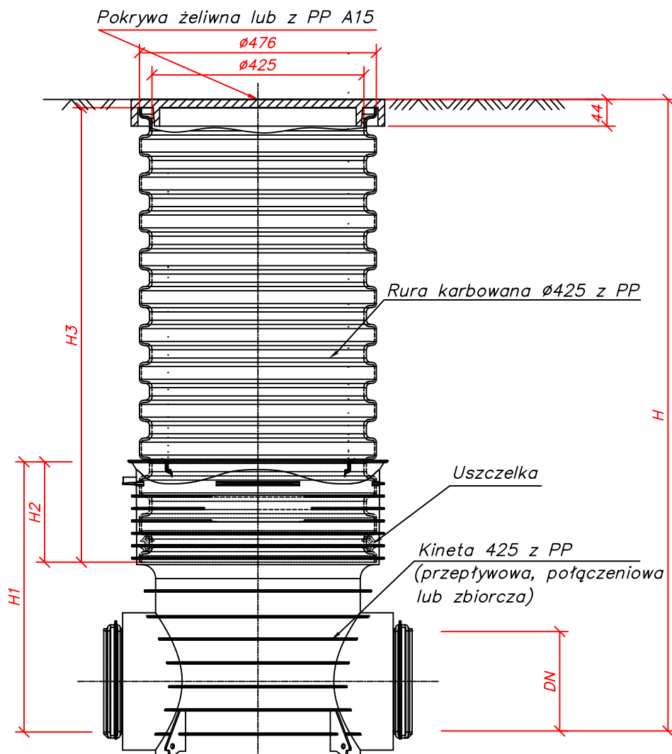
Studzienka inspekcyjna Ø 425 z pokrywą żeliwną lub z PP klasy A15
