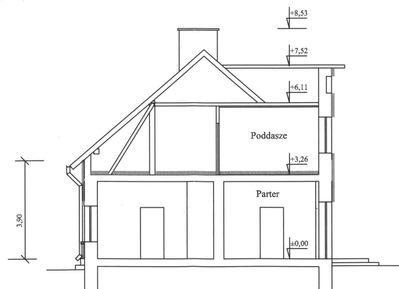
Przekrój A-A
