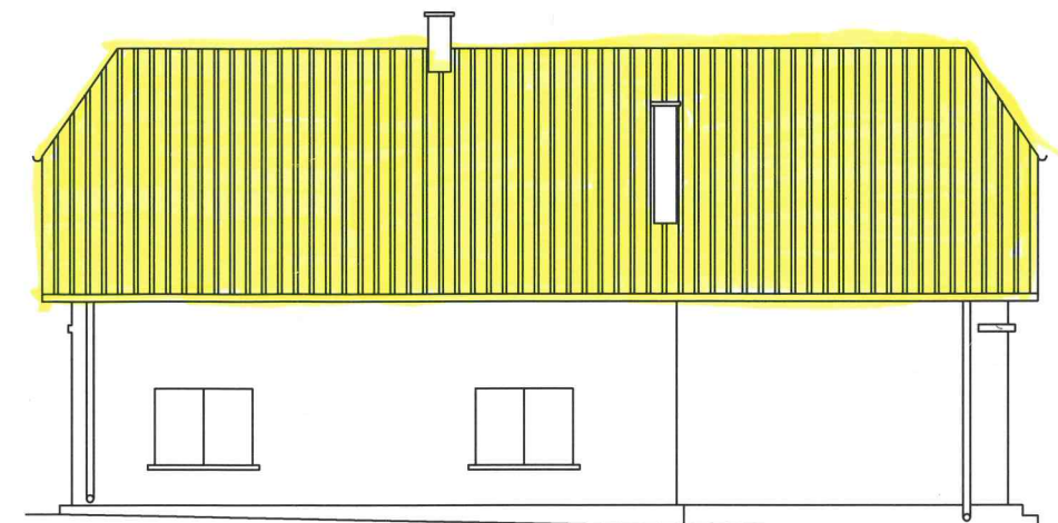
ELEWACJA PÓŁNOCNO-ZACHODNIA
