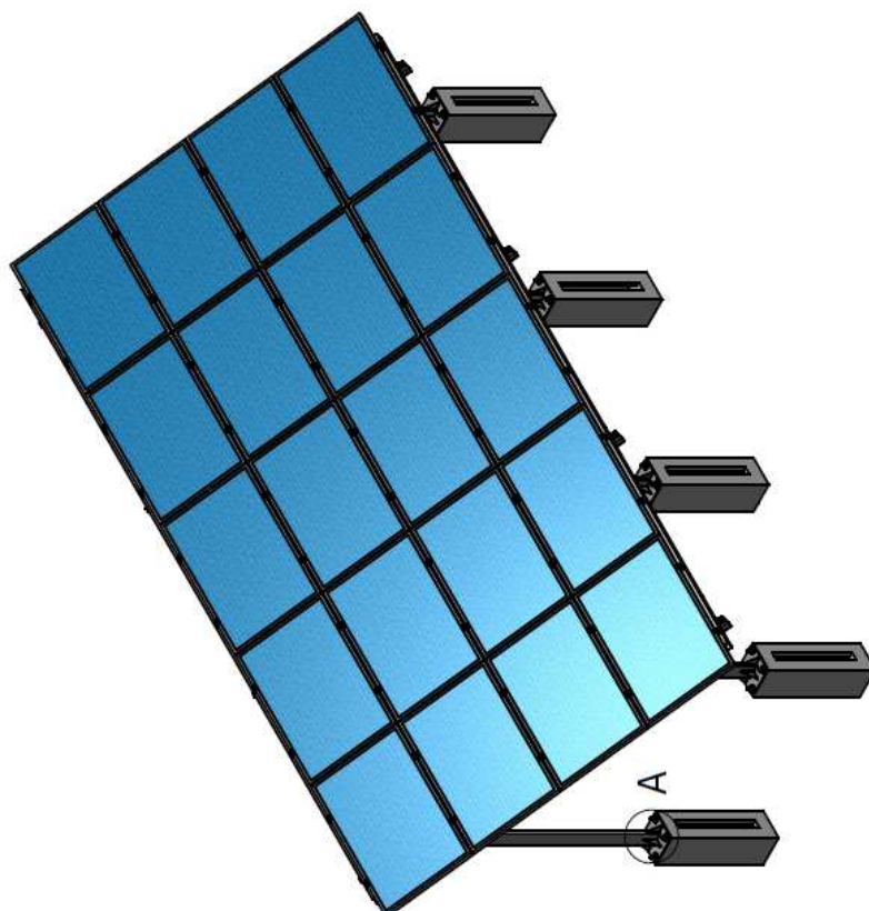
ZAŁĄCZNIK NR 1 - RYSUNEK POGLĄDOWY WYMAGANEJ KONSTRUKCJI WSPORCZEJ . SZKIC ORIENTACYJNY (DLA POTRZEB WYKONANIA PROJEKTU KONSTRUKCYJNEGO)
