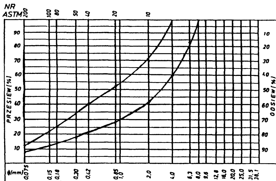
Rys. 3. Krzywe graniczne uziarnienia mieszanki mineralnej 0+8, 0+6,3 mm do warstwy ściernalnej z betonu asfaltowego dla KR 1
