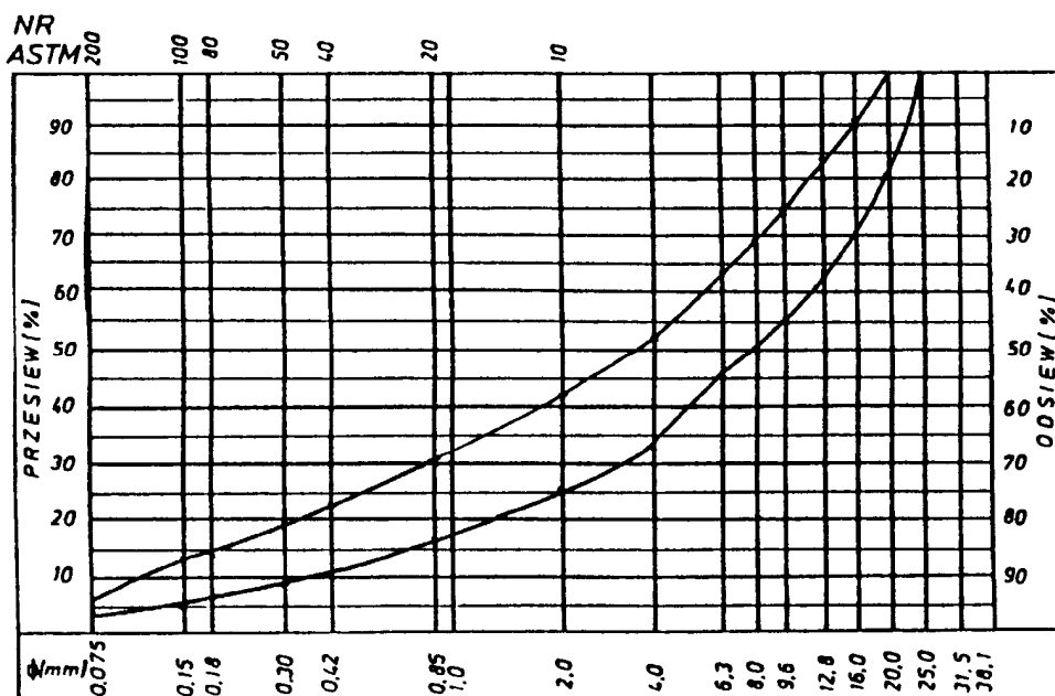
Rys. 10. Krzywe graniczne uziarnienia mieszanki mineralnej 0+12,8 mm do warstwy wiążącej, wyrównawczej i wzmacniającej z betonu asfaltowego dla KR 1
