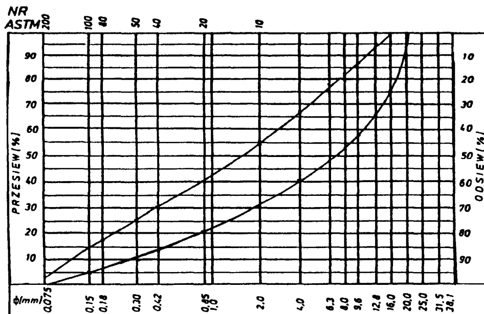
Rys. 8. Krzywe graniczne uziarnienia mieszanki mineralnej 0+20 mm do warstwy wiążącej, wyrównawczej i wzmacniającej z betonu asfaltowego dla KR 1
