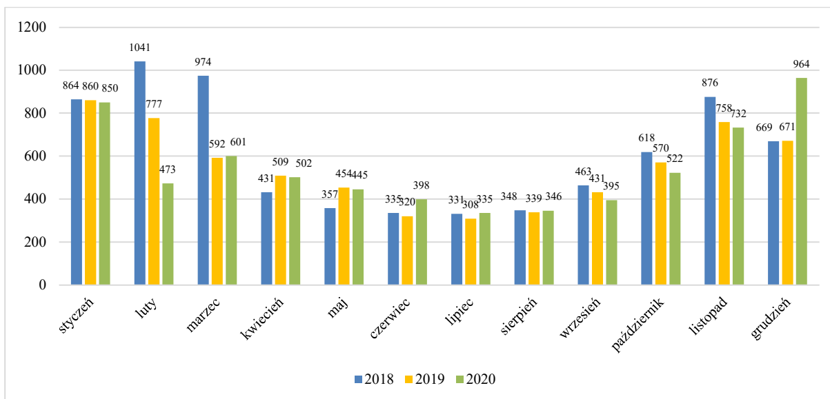
Rysunek 6 Średnie stężenie tlenku węgla na stacji w Lubaniu w latach 2018 – 2020 ( \mu\text{g}/\text{m}^3 )
