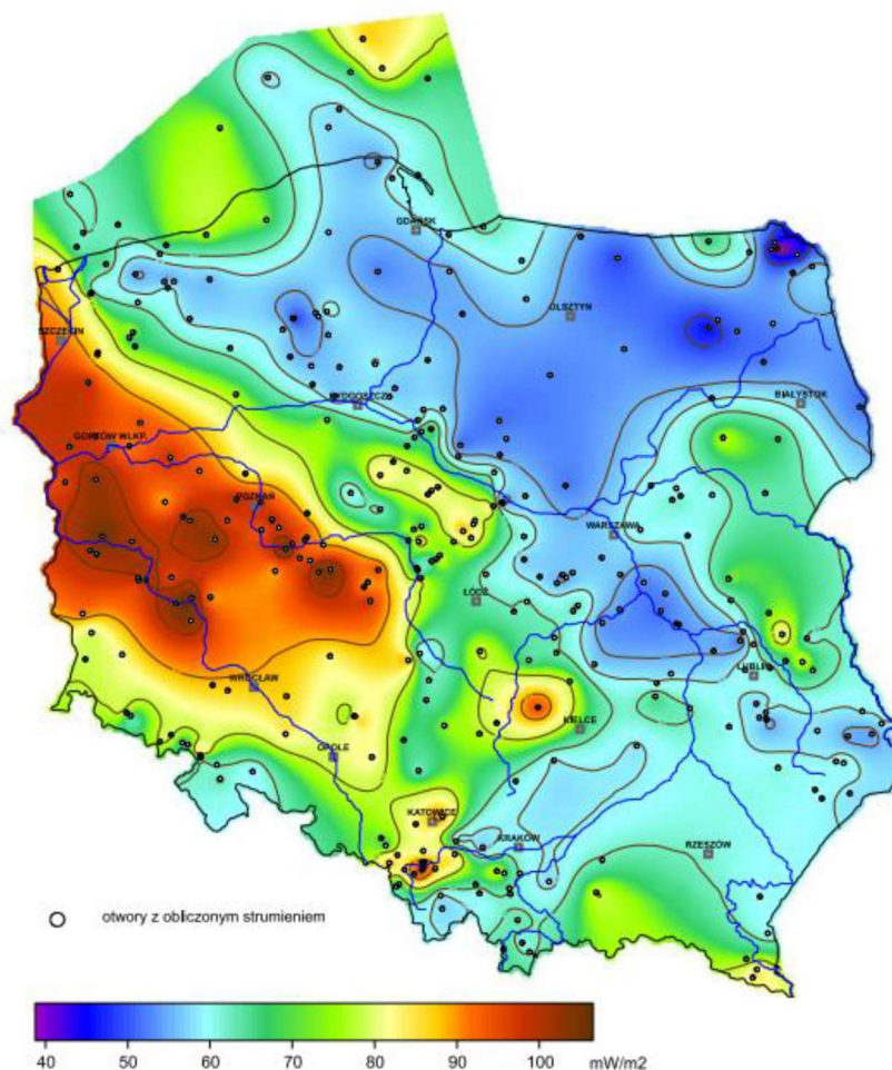
Rysunek 17 Mapa rozkładu gęstości ziemskiego strumienia ciepłego na obszarze Polski Źródło: Szewczyk J., Giętka D., 2009, [za:] Wójcicki A., Sowizdżał A., Bujakowski W., 2013
