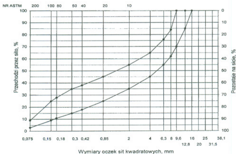
10. Krzywe graniczne uziarnienia mieszanki mineralnej BA od 0 do 12,8 mm do warstwy wiążącej, wyrównawczej i wzmacniającej nawierzchni drogi o obciążeniu ruchem KR1 lub KR2
