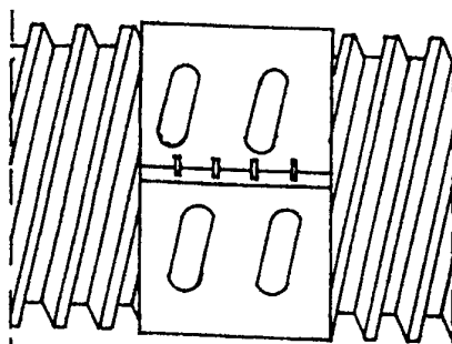
Rys. 4. Ułożenie rur przepustu na słabym gruncie
