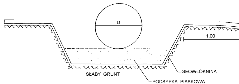
Rys. 4. Ułożenie rur przepustu na słabym gruncie
