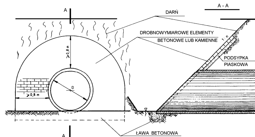
Rys. 6. Przykład umocnienia skarpy przy wlocie przepustu za pomocą drobnowymiarowych elementów z betonowej kostki brukowej lub kamienia
