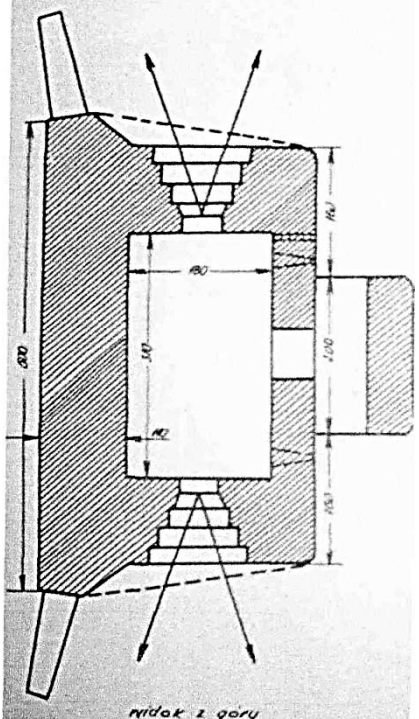
Typ C-2 uzbrojenie 2 ckm załoga 5-8 ludzi
