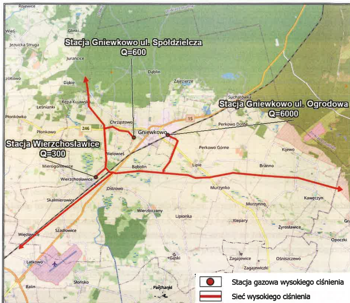
Rysunek 4. Schemat sieci gazowej wysokiego ciśnienia na terenie gminy Gniewkowo
