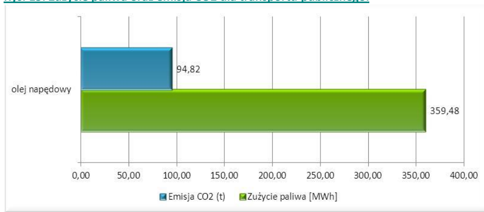
Rys. 15. Zużycie paliwa oraz emisja CO 2 dla transportu publicznego.
