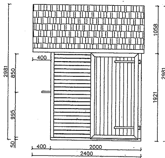
Elewacja boczna
