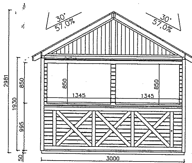
Elewacja frontowa
